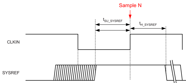
Figure 146. SYSREF Timing (Subclass 1)
