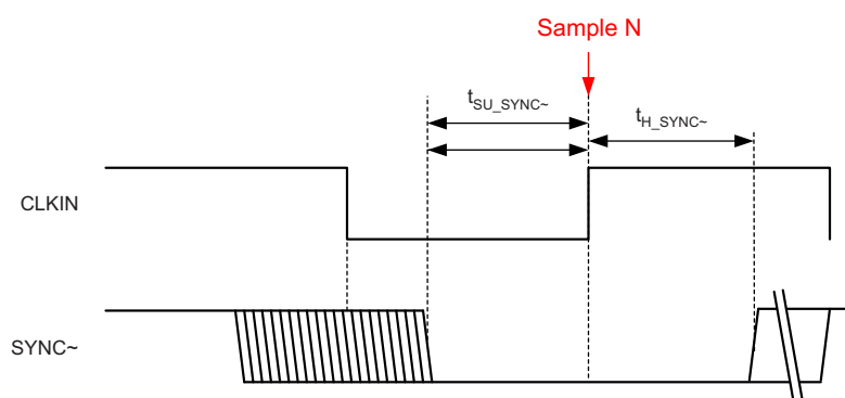
Figure 147. SYNC~ Timing (Subclass 2)
