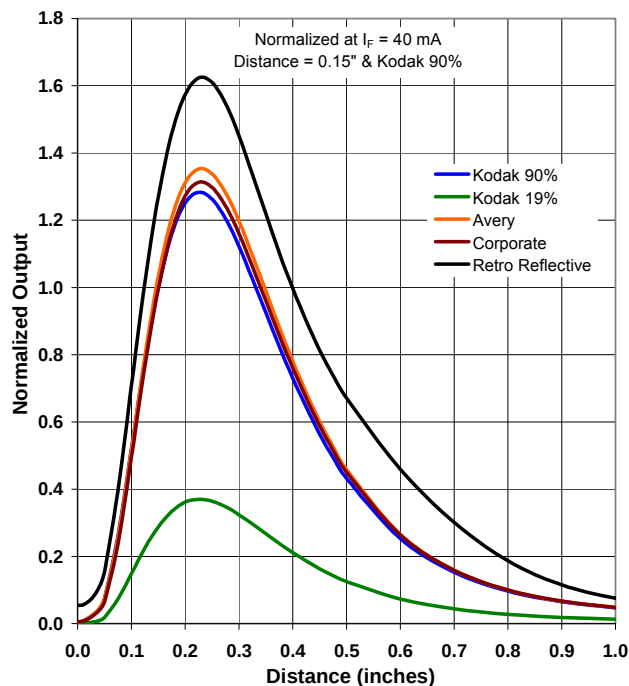
OPB703—Output Distance
