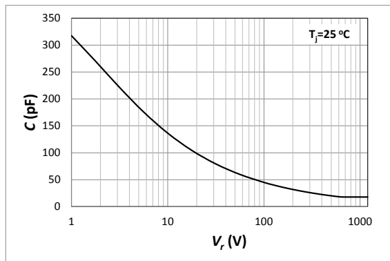
Fig. 5 Capacitance
