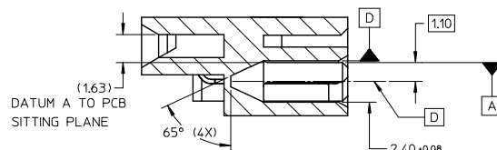
SECTION V-V
