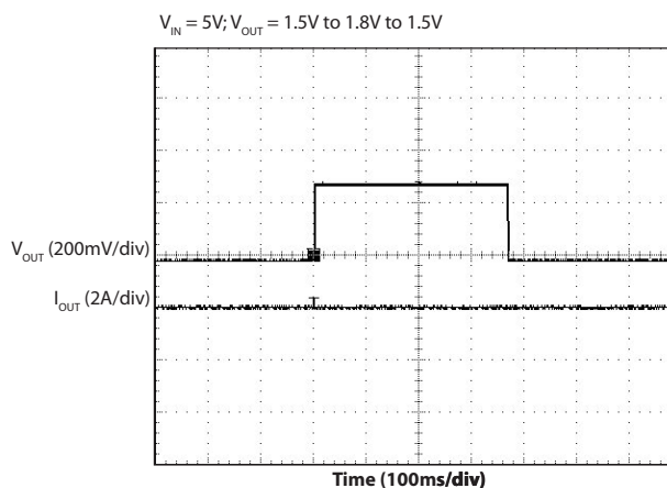
VID Transition — Full Load
