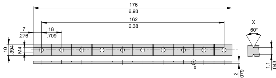
Bus bar Y 303 563 01
