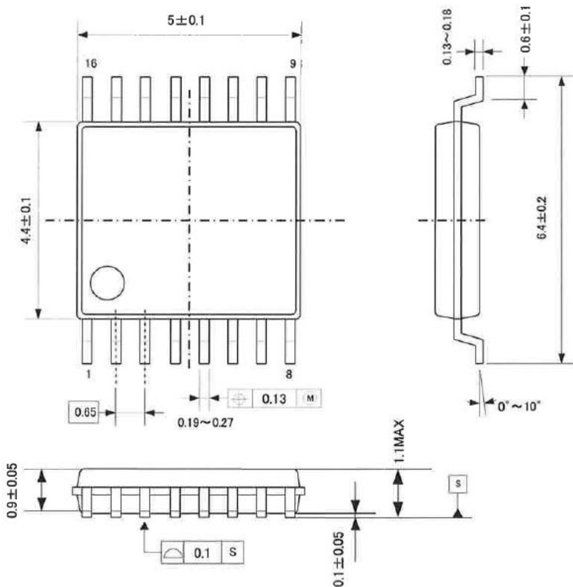
Fig. 18 Outer Dimensions
