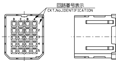
電線挿入側 WIRE SIDE
