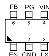
TSOT-23-6/SOT-23-6
