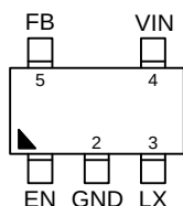
TSOT-23-5
