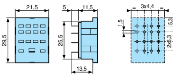
PCB base RTMA4 - 26 532 708
