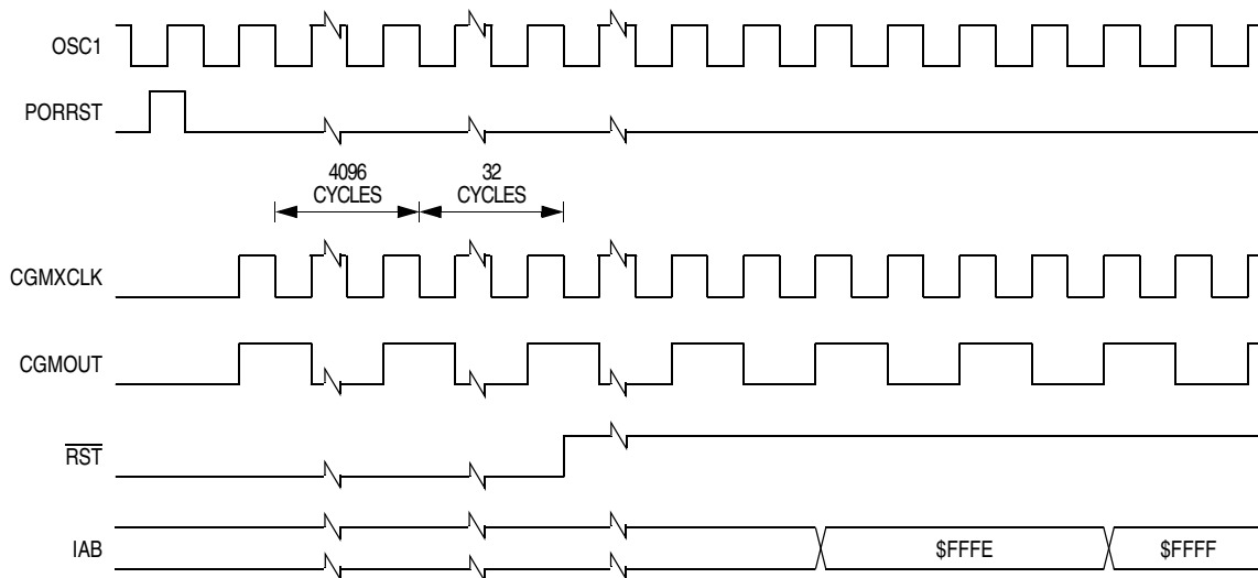
Figure 14-6. POR Recovery
