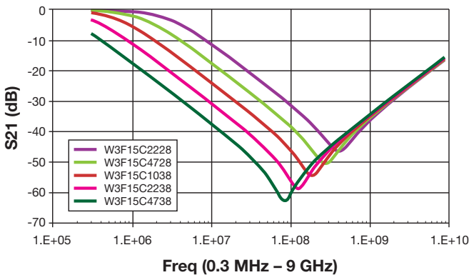
S21 1206 – 50V
