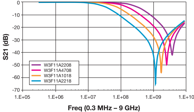
S21 1206 – 100V
