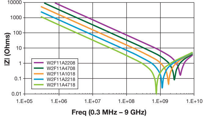
IMPEDANCE 0805 – 100V
