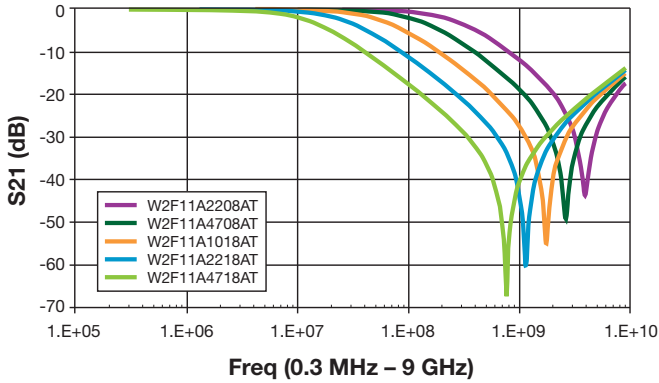
S21 0805 – 100V
