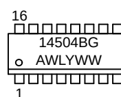
SOIC-16
