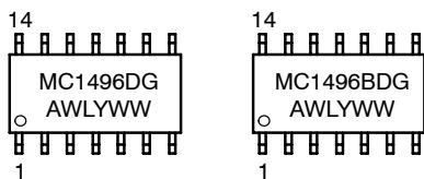
SOIC-14 D SUFFIX CASE 751A
