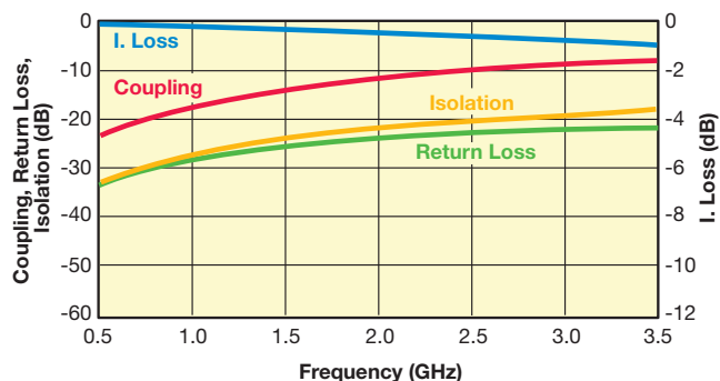
CP0603A****AS
