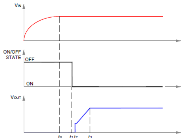
Fig. H: Startup scenario #3.
