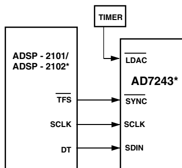
Figure 11. AD7243-ADSP-2101/ADSP-2102 Interface
