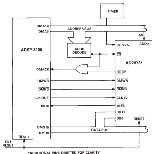
Figure 18. AD7878-ADSP-2700 Interface
