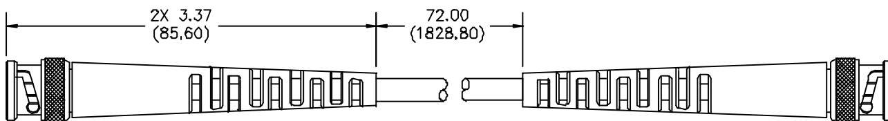
TRUE 75 BNC CABLE, BLUE (MODEL 6510-V-72-6)
