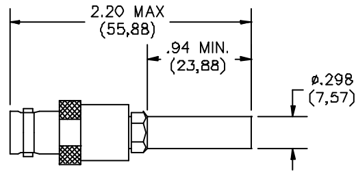
MINI WECC/BNC ADAPTER (4X MODEL 6519)
