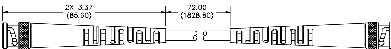
TRUE 75 BNC CABLE, RED (MODEL 6510-V-72-2)
