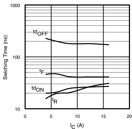
Fig. 13 - Typ. Switching Time vs. I_C T_J = 150^\circ\text{C} ; L=1.1\text{mH} ; V_{CE}=400\text{V} R_G=50\Omega ; V_{GE}=15\text{V}
