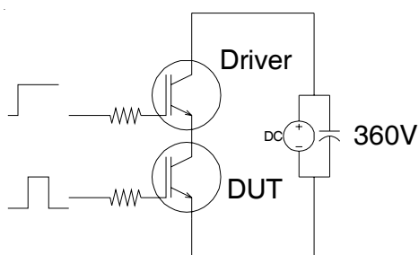
Fig.C.T.3 - S.C.SOA Circuit
