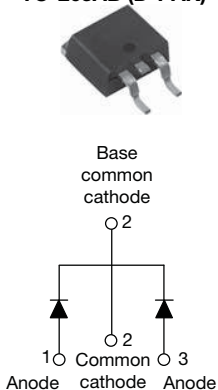
VS-MBRB25..CTPbF
