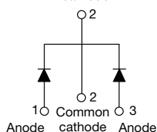
VS-48CTQ060SPbF
