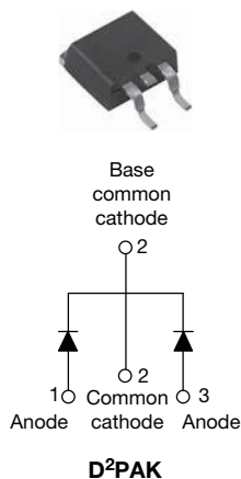
VS-MBRB20..CTPbF
