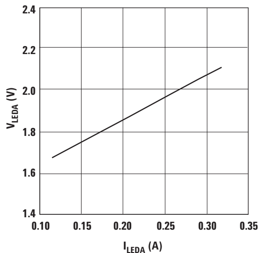
Figure 10. V_{LEDA} vs I_{LEDA} .
