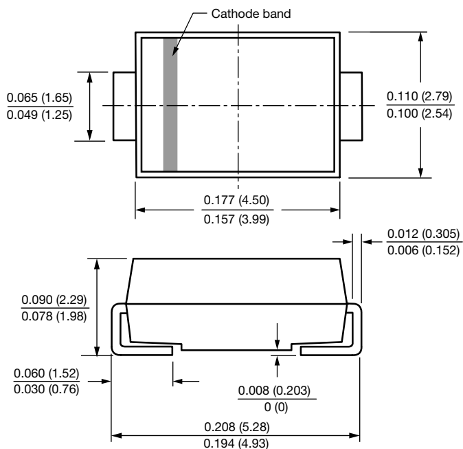
DO-214AC (SMA)
