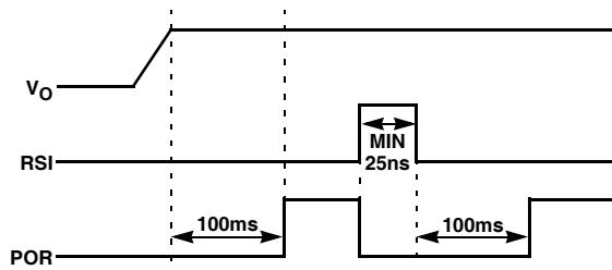
FIGURE 14. RSI & POR TIMING DIAGRAM
