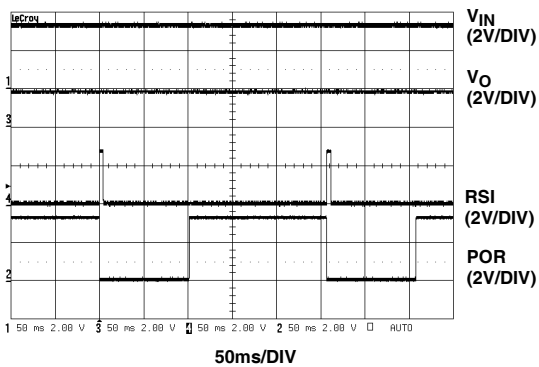
FIGURE 9. POR FUNCTION
